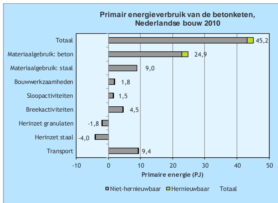
Figuur 13 Primair energieverbruik van de betonketen (exclusief gebruik van bouwwerken), totaalgebruik beton in 2010
