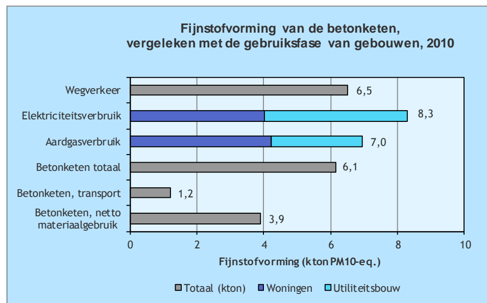
Figuur 18 Fijnstofvorming van de betonketen vergeleken met gebruik van gebouwen en wegen, 2010
