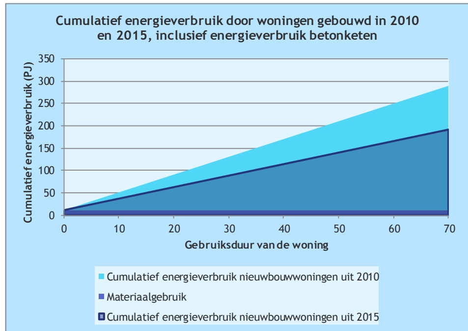
Figuur 21 Verschil in cumulatief energieverbruik door woningen gebouwd in 2010 (EPC 0,8) en 2015 (EPC 0,4)
