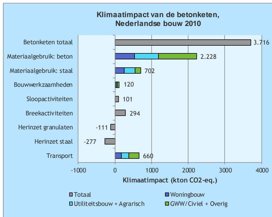
Figuur 11 Klimaatimpact van de betonketen, uitgesplitst naar toepassingsgebied
