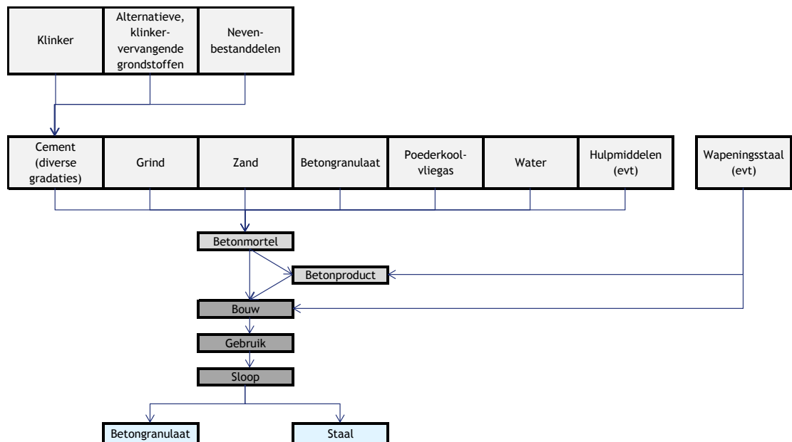
Figuur 3 Schematisch overzicht van ketenfasen voor beton- en wapeningsstaal
